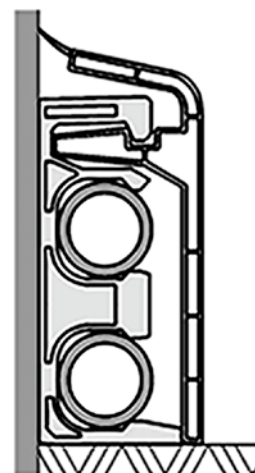
Řez zalištovaným potrubím
